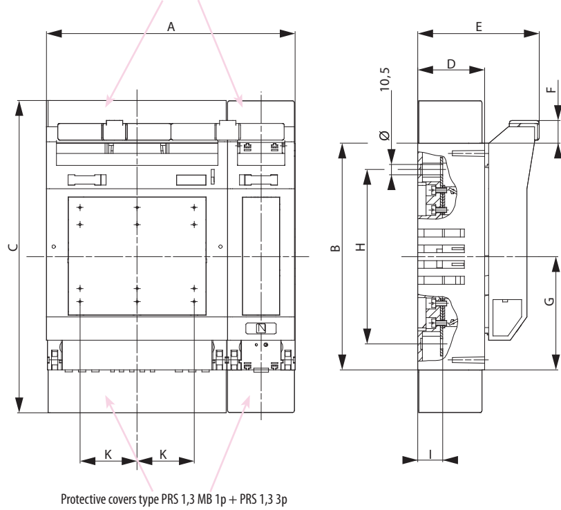
Protective covers type PRS 1,3 MB 1p + PRS 1,3 3p
