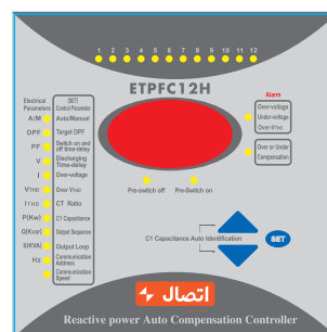
رگولاتور خازنی
