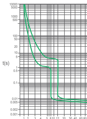
I/I_n C curve
