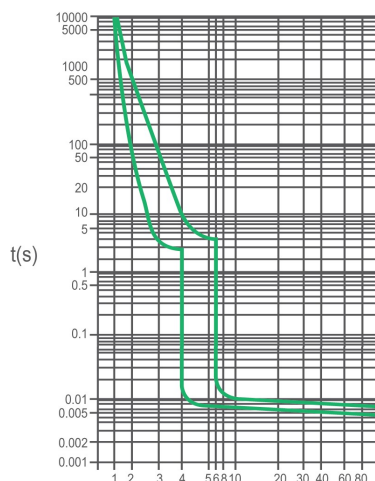
I/I_n B curve
