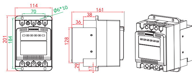
مدل S تا ۵۰ کیلووار
